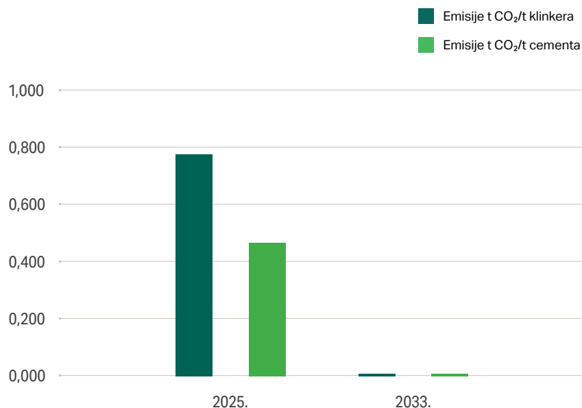
NEXE CO 2 emisije
