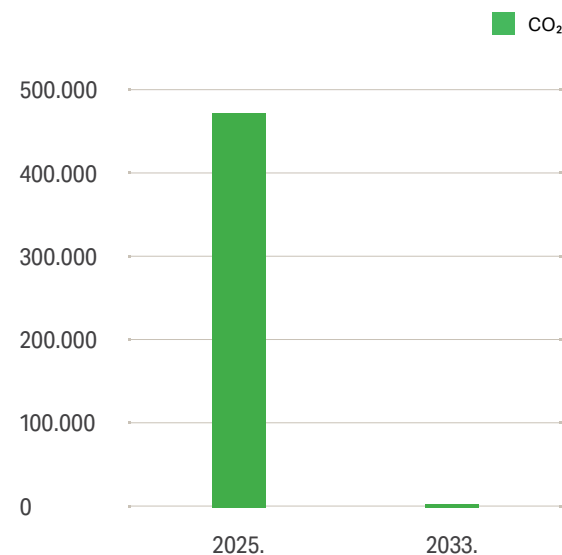
NEXE d.d. CO 2 emisije (fosilne)
